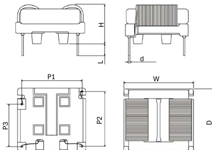
SQ15H
