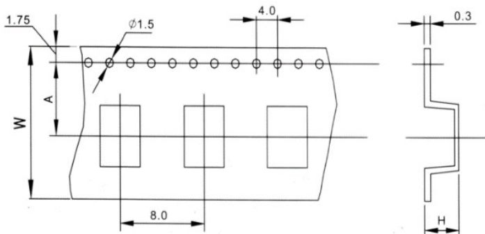
●テープ寸法 / Taping dimension (mm)
