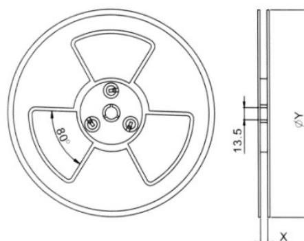
●リールサイズ / Reel size (mm)
