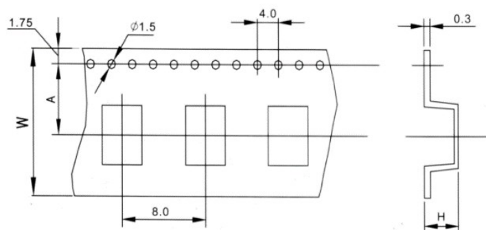
●テープ寸法 / Taping dimension (mm)
