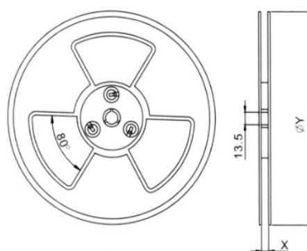
●リールサイズ / Reel size (mm)
